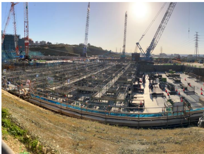
写真⑪ (躯体工事 B棟 基礎・地中梁躯体工事状況)
