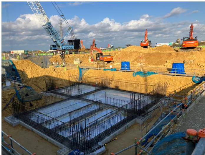
写真⑪(土工事 B棟 ピット部埋戻し)
