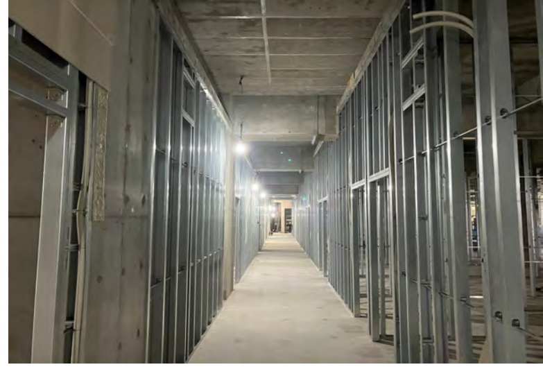
写真⑫ (B棟 金属工事 3階壁軽量鉄骨下地施工状況)
