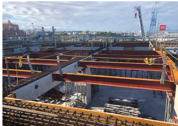
写真⑩(A棟 鉄骨工事 8階梁架設状況)
