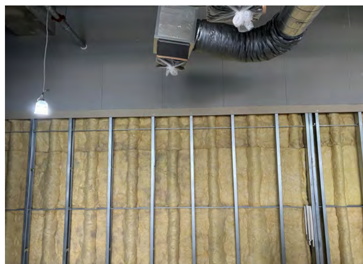
写真⑫ (B棟 金属工事 2階壁軽量鉄骨下地施工状況)
