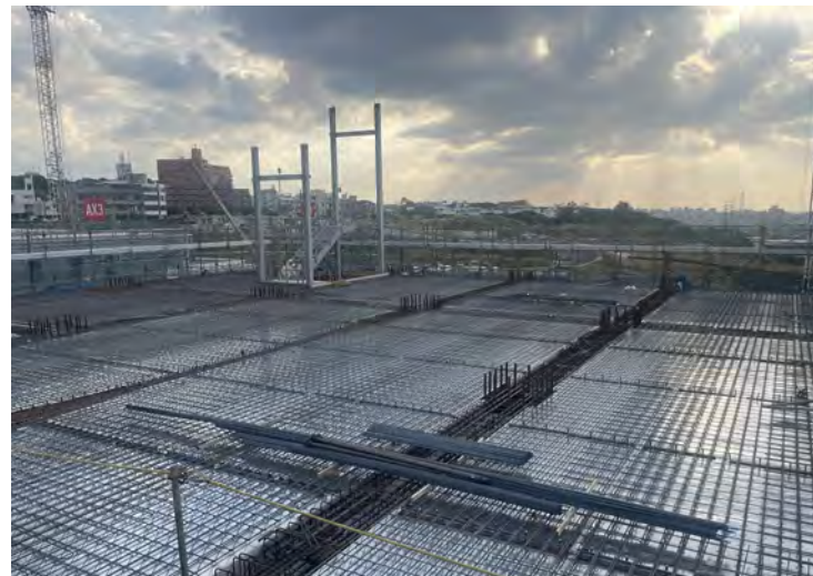
写真⑩(A棟 鉄骨工事 7階デッキスラブ 敷設状況)
