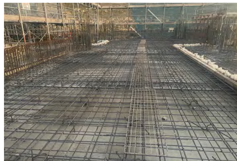
写真⑭(D棟 鉄筋工事 B1階床配筋状況)
