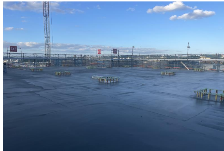
写真⑩(A棟 コンクリート工事 5階床コンクリート打設状況)
