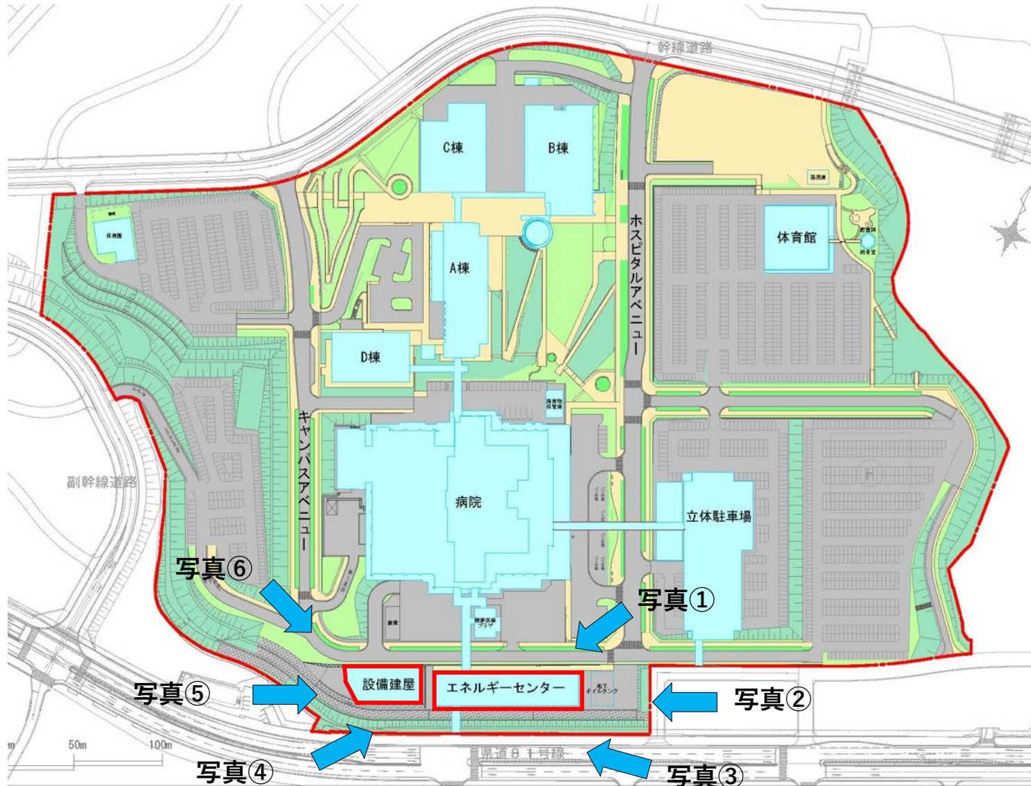
配置図
