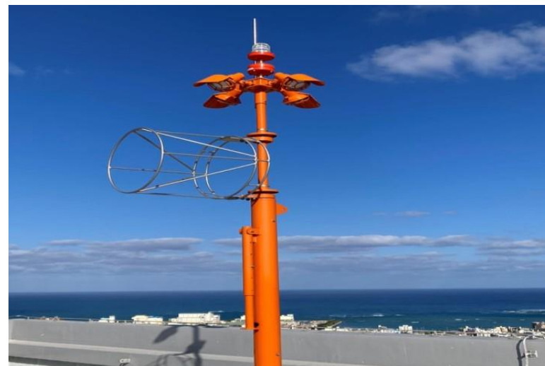
写真⑯(電気工事 風向指示器設置状況 (屋上))
