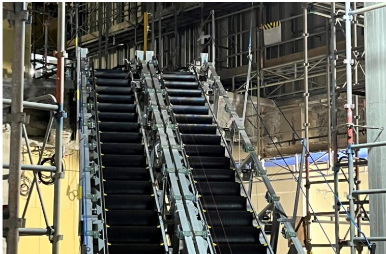
写真⑪(昇降設備工事 エスカレータ施工状況)
