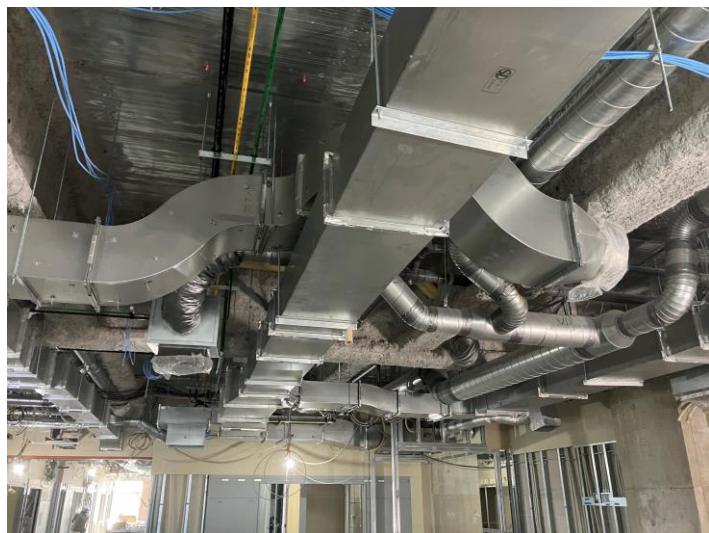
写真⑬(機械工事 8階スタッフステーション 天井内吊込状況)
