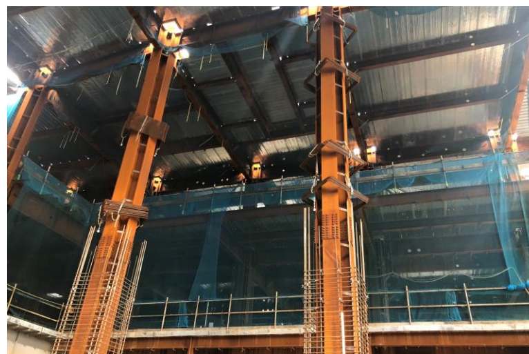
写真⑫(鉄骨工事 2階エントランスホール施工状況)
