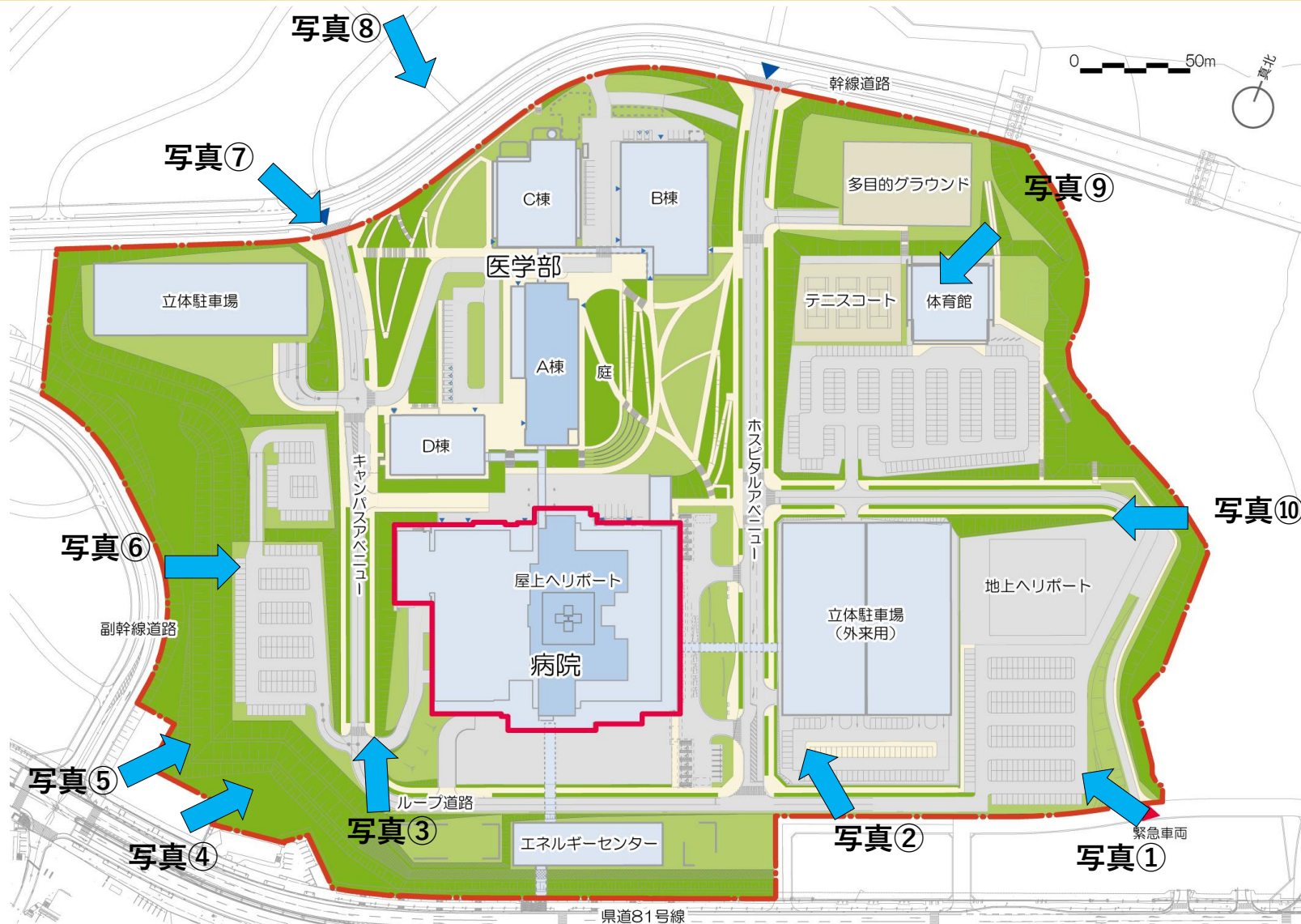
配置図
