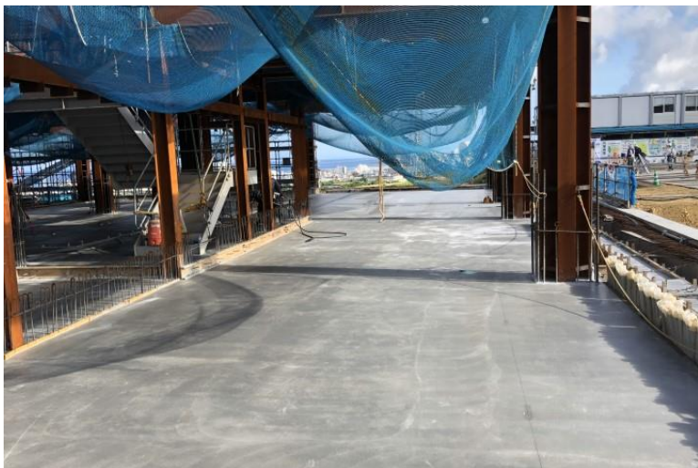
写真⑪(コンクリート工事 2階床コンクリート施工状況)
