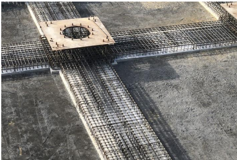
写真⑪(鉄筋工事 1階基礎梁配筋施工状況)
