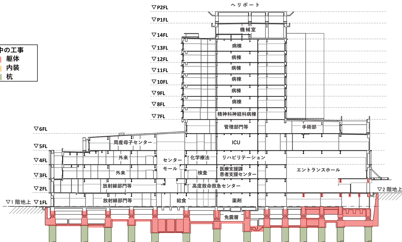
断面図
