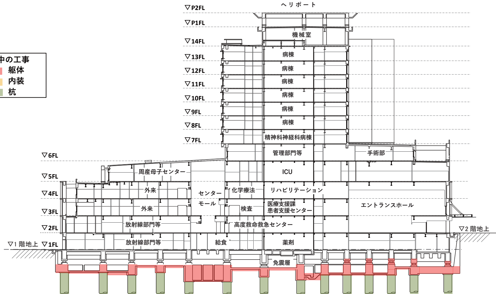
断面図
